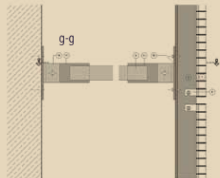
Detail Fassadenstoß
