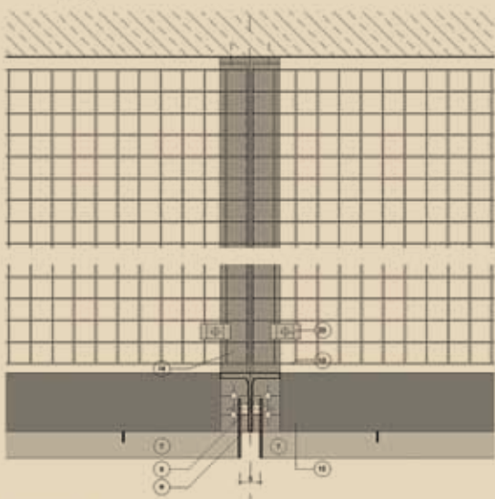
Schnitt f-f
