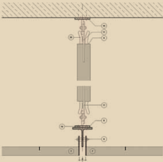
Schnitt g-g
