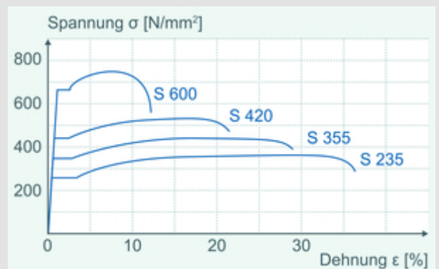
Abb. 2: Spannungs-Dehnungsdiagramm
