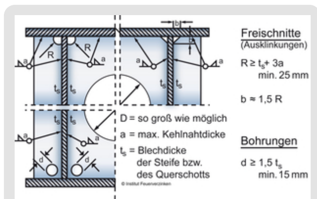
Abb. 7: Freischnitte an Schotten von Hohlbauteilen nach DAST-Richtlinie 022
