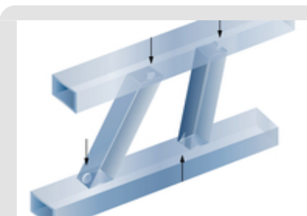
Abb. 4: Möglichkeiten der Entlüftung von Fachwerkträgern nach DIN EN ISO 14713-2.
