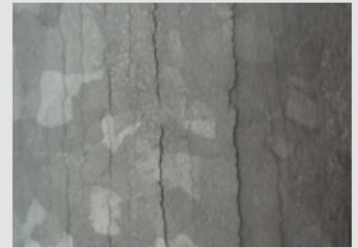
Abb. 4 Rissiger, abplatzender Zinküberzug an einer Stahlstütze infolge eines Frostschadens
