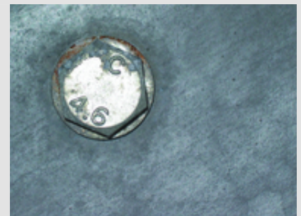
➔ Abb. 3: Falsch - Galvanisch verzinkte Schraube mit beginnendem Rotrost in feuerverzinkter Stahlkonstruktion.
