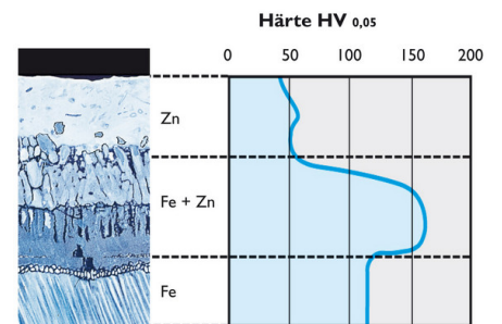
Abb. 2: Härteverlauf eines Zinküberzuges
