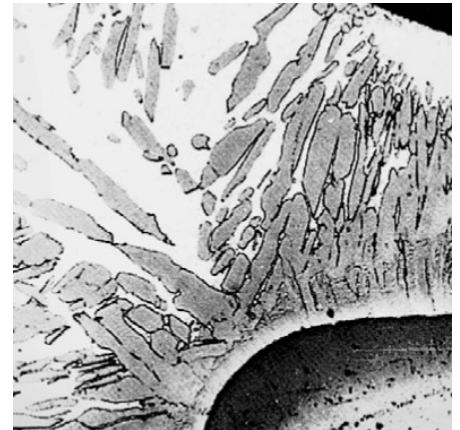
Abb. 4: Kantenflucht tritt beim Feuerverzinken nicht auf.
