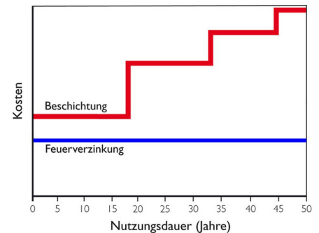
Abb. 6: Die Feuerverzinkung verursacht keine Folgekosten und ist zumeist bei den Erstkosten günstiger.
