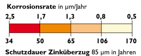
Abb. 1: Zinkkorrosionskarte des Umweltbundesamtes: Schutzdauer eines Zinküberzuges mit 85 µm Schichtdicke
