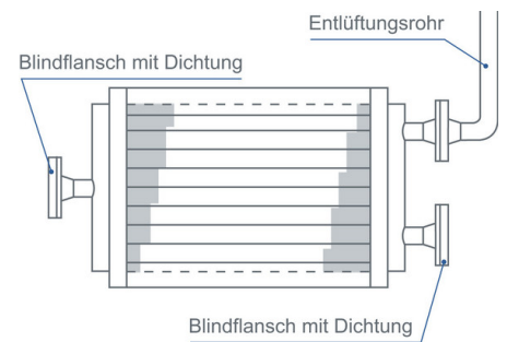
Abb. 4: Zusatzmaßnahmen zum Abdichten und Entlüften bei der "Nur-Außenverzinkung".
