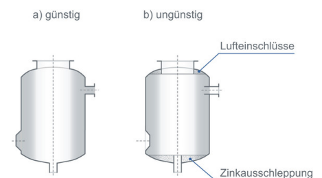
Abb. 2: Anschlüsse, Flansche und Stutzen sollten möglichst groß sein und bündig mit der Behälteroberfläche abschließen.
