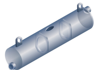
Abb. 3: Große und schwere Behälter sollten möglichst mit Aufhänge-Ösen versehen werden.
